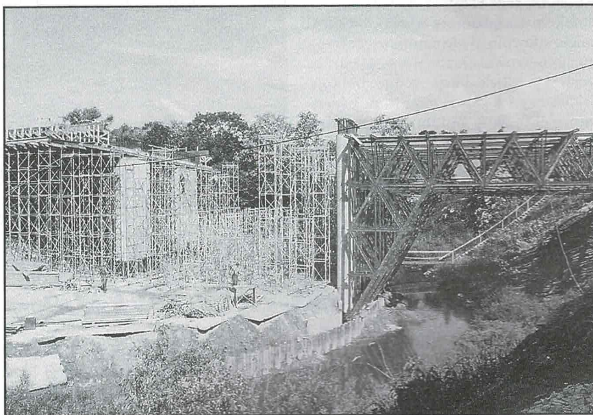
Budowa mostu na "Zielonce"
