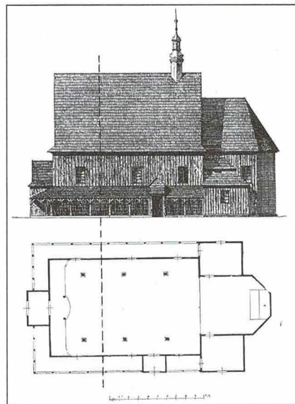
Widok i plan kościoła w Tymowej wg. F. Kopera i L. Lepsi, Kościół drewniane w Galicji Zachodniej , Kraków 1916.
