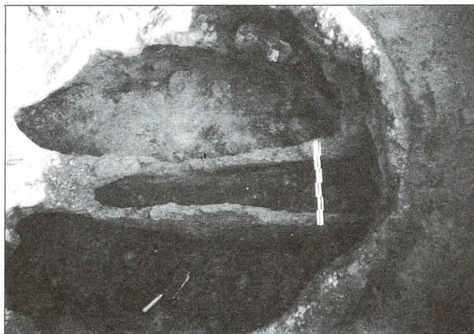
Przegroda paleniska pieca z glinianą rurą.
