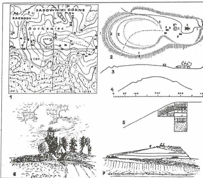
Dokumentacja grodziska na Bocheńcu z 1947 r. (wg G. Leńczyka) 1-lokalizacja, 2-plan grodziska, 3,4-przekroje przez wały, 5-profil i rzut wykopu z układem belek konstrukcji wału, 6-wał zaporowy od wschodu, 7-panorama wzgórza
